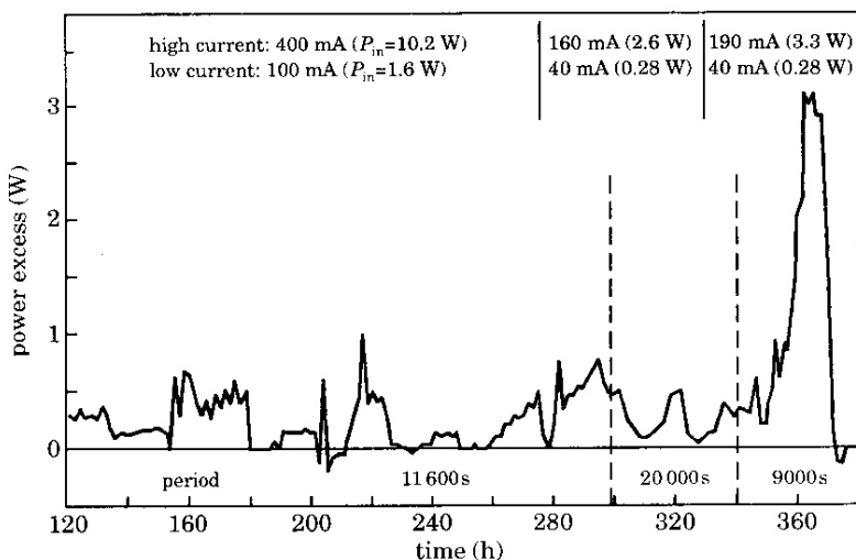
Fig. 5 - Un grafico della potenza in eccesso in funzione del tempo, ottenuto nel secondo dei tre esperimenti realizzati nel 1992
