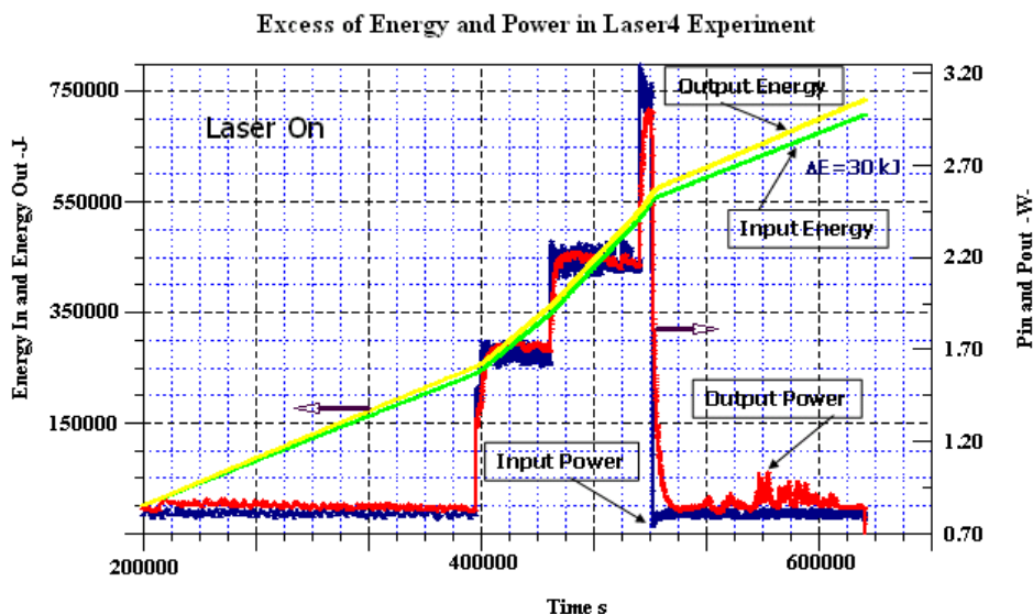
Fig. 4 - Andamento della potenza e dell'energia in ingresso ed in uscita durante l'esperimento Laser4
