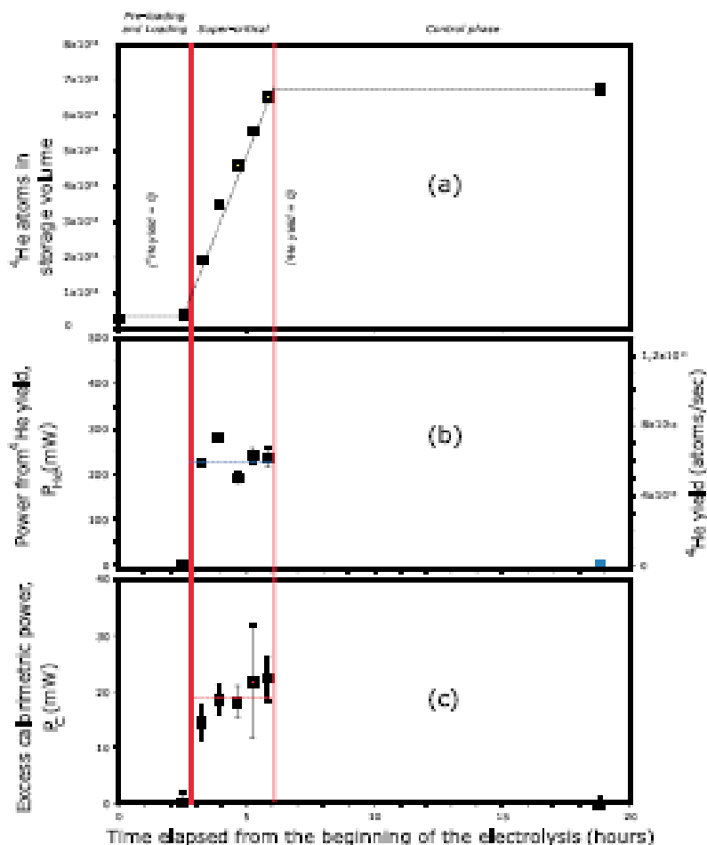
Fig. 1 - (a) Contenuto di ^4\text{He} nella miscela di gas provenienti dalla cella elettrolitica
